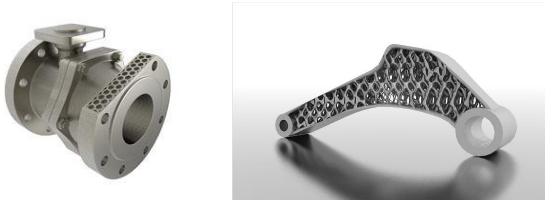
1. ábra Példa rácsszerkezettel könnyített gépipari gyártmányokra
