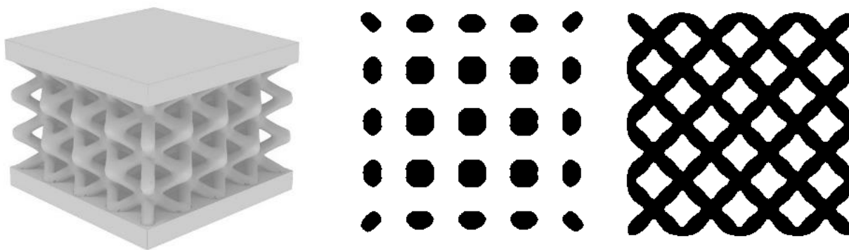
5. ábra Rácsszerkezettel könnyített 3D modell és annak jellemző keresztmetszetei
