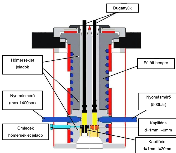
2. ábra. Mérőhenger elvi vázlata
